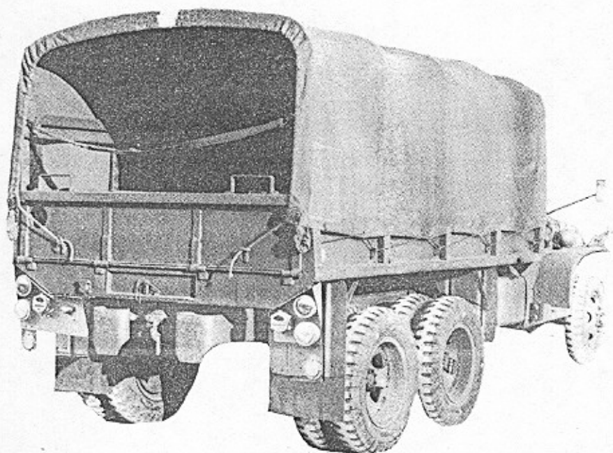
2½ t GMC, 6x6, CCKW 353, last Set skråt bagfra, højre side.
